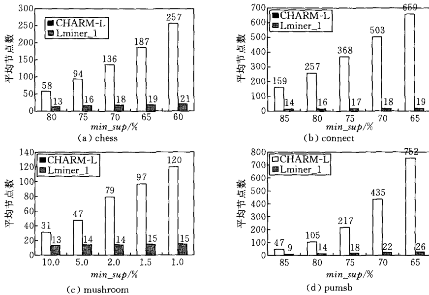
图8 考察每个收缩对时需访问的平均节点数
