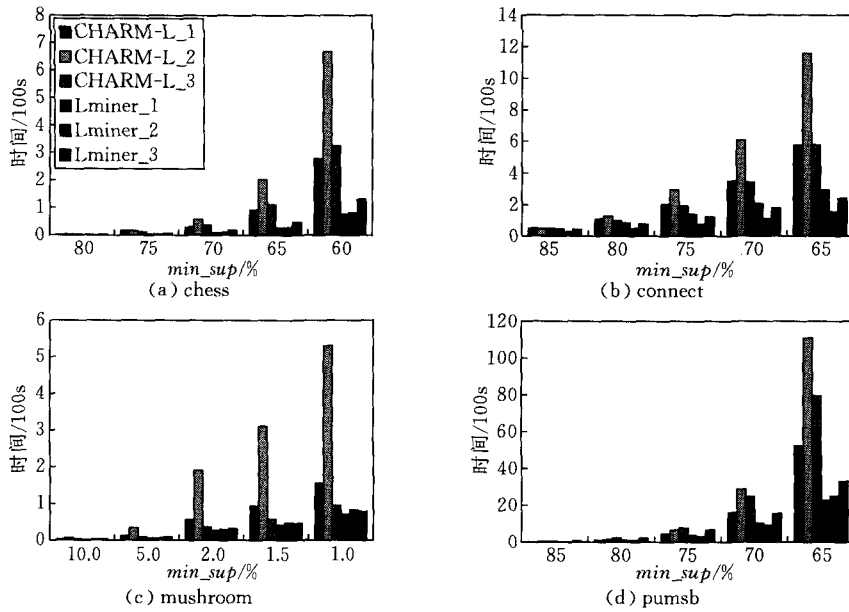
图7 表3中数据集在不同 min_sup 下的格挖掘速度
